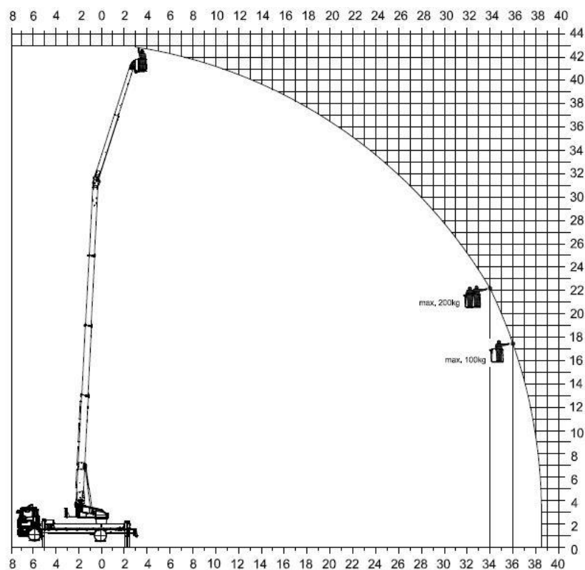
Abb. 4-4 Arbeitsbereich Hubarbeitsbühnenbetrieb K 1000 RSX (Klappspitze einfach ausgefahren)
