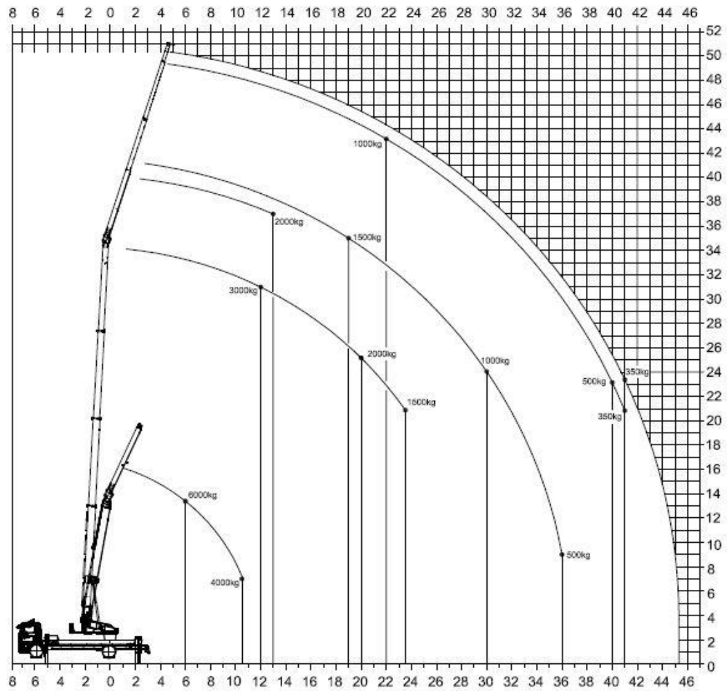
Abb. 4-2 Arbeitsbereich Kranbetrieb K 1000 RSX (Traglastdiagramm)
