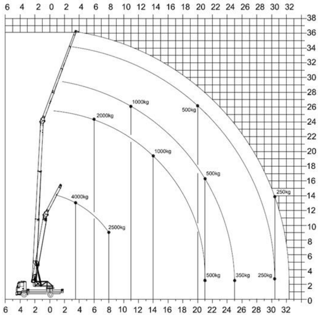
Abb. 4-2 Arbeitsbereich Kranbetrieb K 30-37 TSR (Traglastdiagramm, maximale Abstützbreite)
