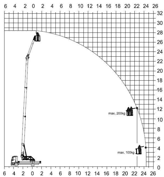
Abb. 4-3 Arbeitsbereich Hubarbeitsbühnenbetrieb K 30-37 TSR (Normalbetrieb)
