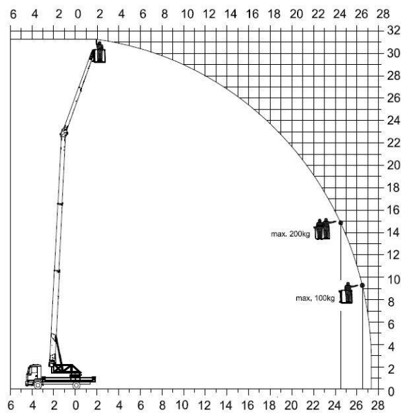
Abb. 4-4 Arbeitsbereich Hubarbeitsbühnenbetrieb K 30-37 TSR (Klappspitze einfach ausgefahren)
